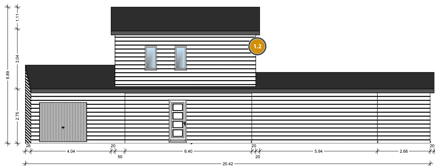
FACADE NORD
