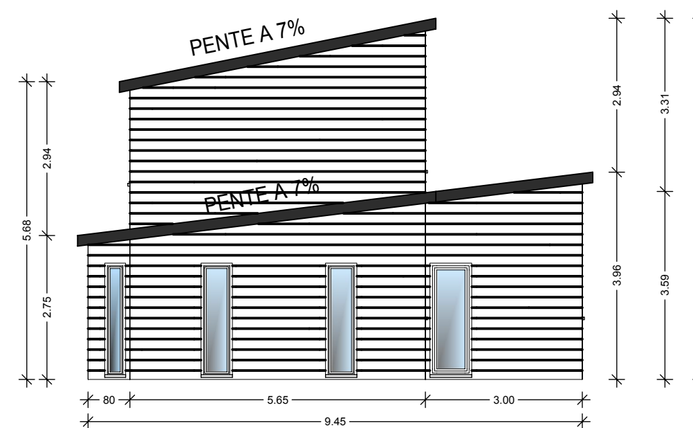
PIGNON OUEST
